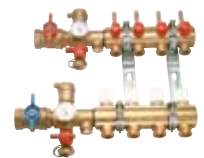
Colectores pre-ensamblados
